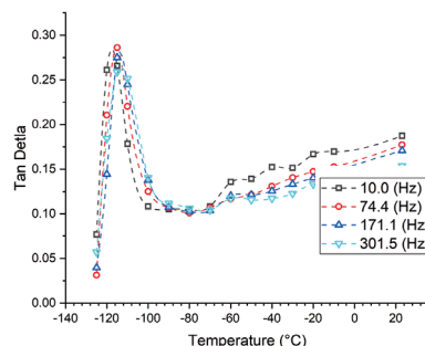
nanoDMAを用いたポリジメチルシロキサンフィルムの動的粘弾性評価、-110°C付近にtan δのピーク(≒ガラス転移点)を確認
