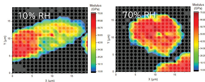
ガラスファイバー充填ナイロン66の弾性率評価、湿度の違いによるガラスファイバー近傍のナイロン66の機械的特性の変化を調査
