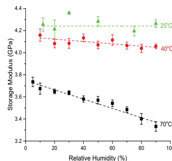
セルロースアセテートの温湿度依存性評価、70°Cでは高湿度になると弾性率が低下
