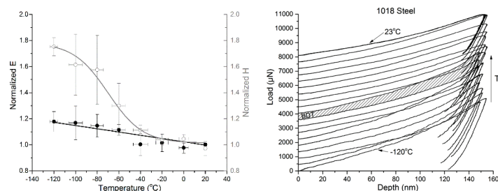
1018炭素鋼の脆性延性遷移の評価、冷却に伴い脆化が生じ、硬さが増加
