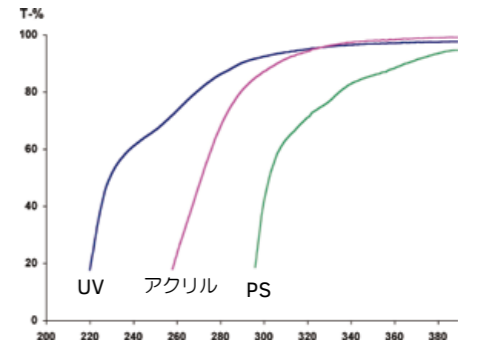
【 各材質の波長ごとの光透過性 】
